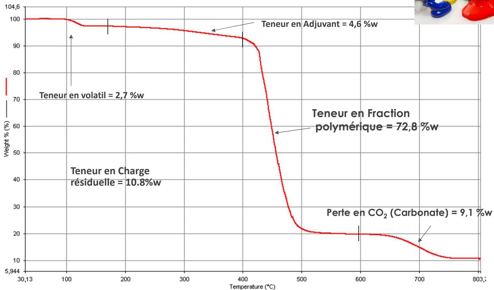
Thermogramme TGA d'une peinture Acrylique sans solvant
